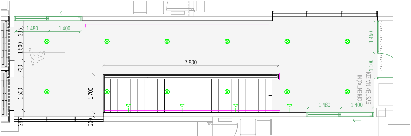
PŮDORYS 3 NP
