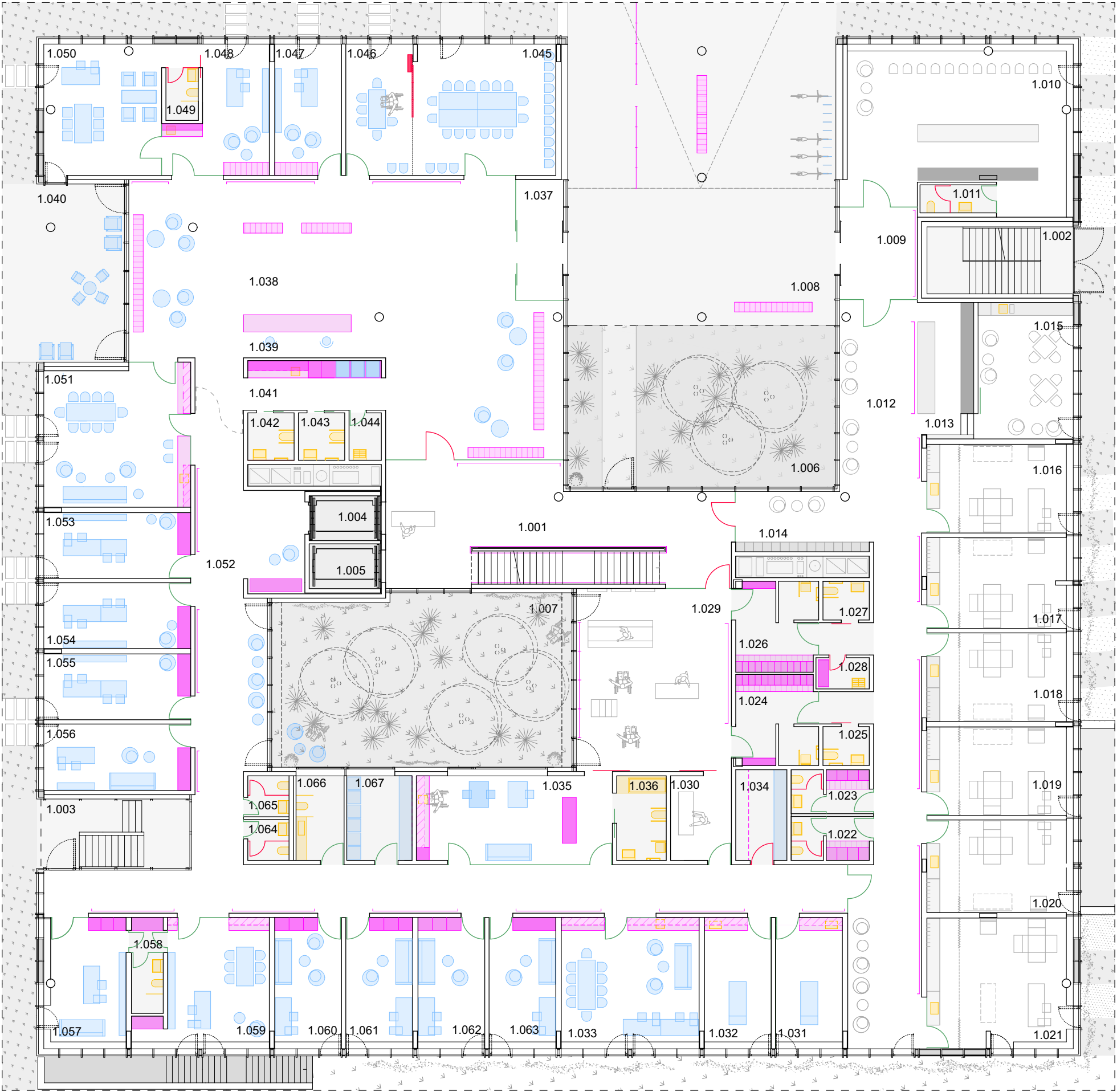
TABULKA MÍSTNOSTÍ 1NP
