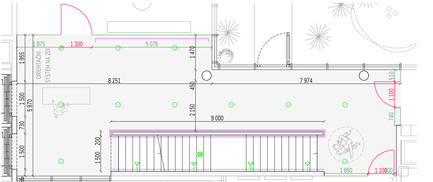
PŮDORYS 1 NP
